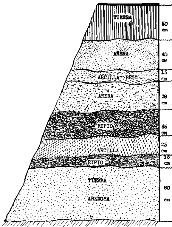
Fig. 9. Corte estratigráfico levantado en la barranca del Río Seco Morado, zona del Paradero Limeño. Podrá apreciarse en este esquema la existencia de estratos arcillosos, arena, ripio, etc., de donde los indígenas habrán sacado dichos ingredientes, para la fabricación de sus recipientes cerámicos.
